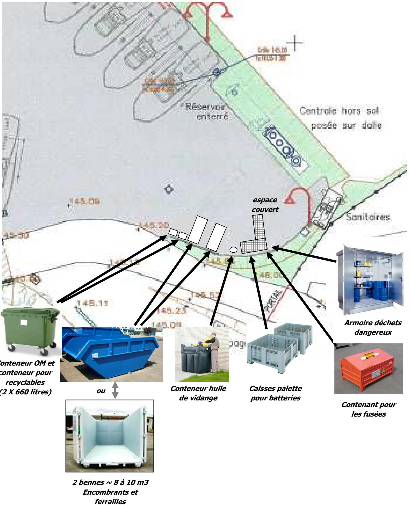
SCHEMA DE PRINCIPE DE L'IMPLANTATION DE LA DECHETTERIE D'APRES LE PLAN DE LA CNR Echelle à vérifier
